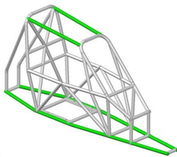
Figura 13 - Desenho 279B-6
