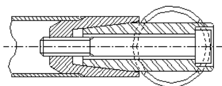
Figura 20 - Desenho 253-39
