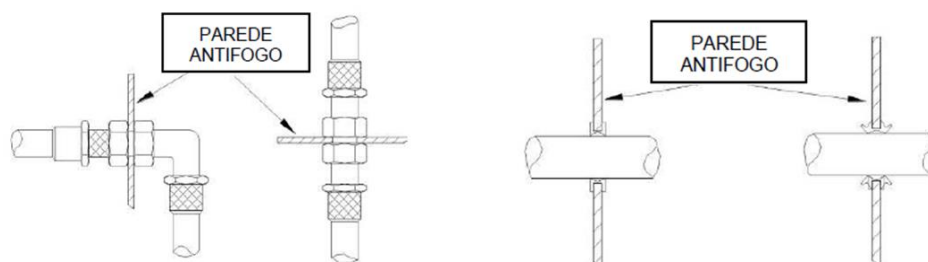
Figura 28 - Furações na parede antifogo - Anexo J - 253-59/60
