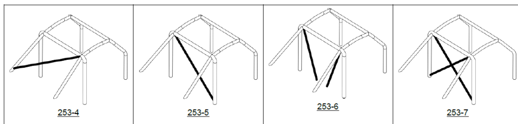
Figura 26 - Tipos de diagonais aceites - Anexo J - 253-4/5/6/7
