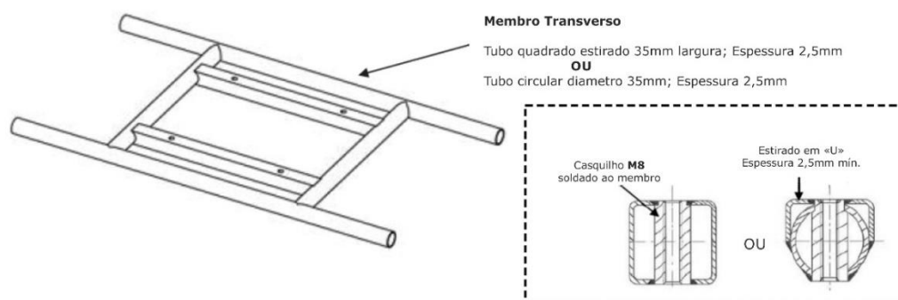
Figura 5 - Construção "D"
