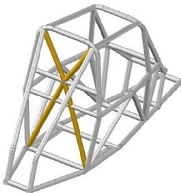
Figura 21 - Desenho 279B-9
