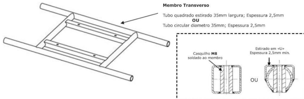
Figura 5 - Construção "D"
