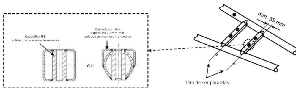
Figura 4 - Construção "C"
