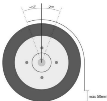
Figura 9 - Esquema de montagem dos guarda-lamas
