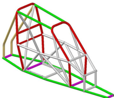
Figura 17 - Desenho 279B-1
