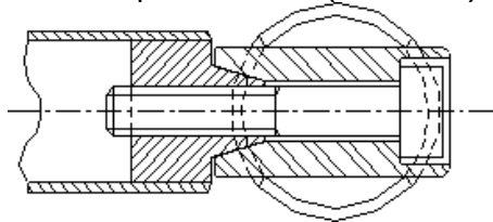
Figura 19 - Desenho 253-38
