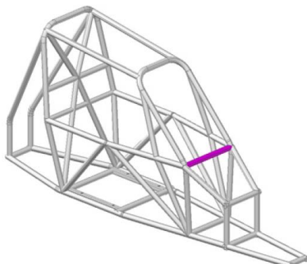
Figura 24 - Desenho 279B-12
