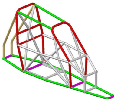
Figura 17 - Desenho 279B-1
