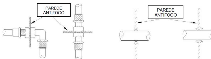
Figura 28 - Furações na parede antifogo - Anexo J - 253-59/60
