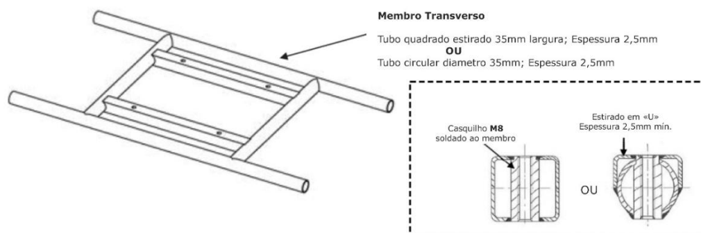
Figura 5 - Construção "D"
