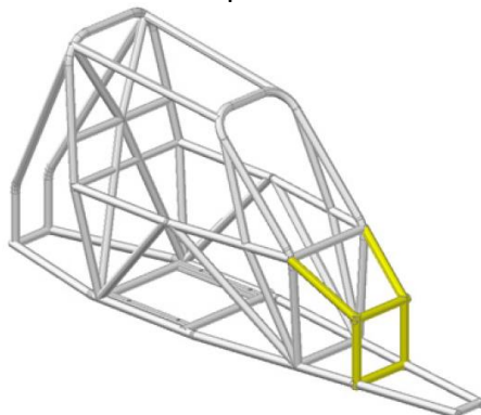
Figura 25 - Desenho 279B-13
