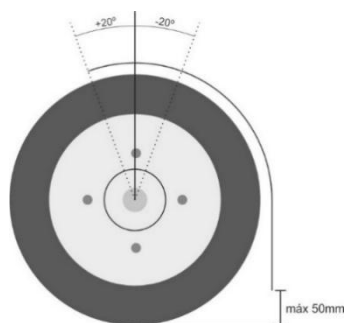
Figura 9 - Esquema de montagem dos guarda-lamas
